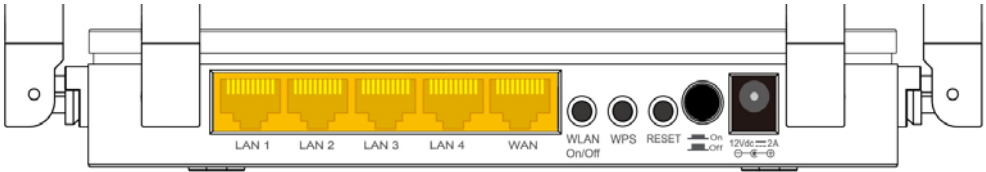
Figuur 1: Aansluitingen router achterzijde
