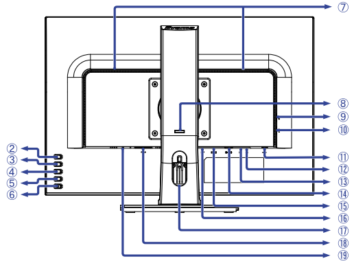
<Achterkant>
