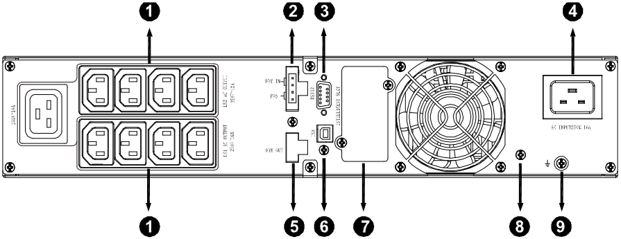
Panneau arrière pour modèle 3000 VA standard
