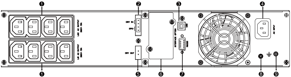
1000VA /1500VA/2000VA Standard & 1000VA /1500VA Super charger model rear panel
