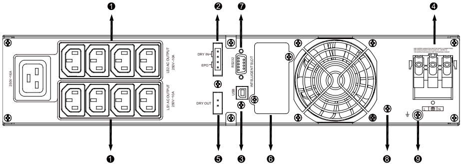
Panneau arrière pour modèle 3000 VA à autonomie prolongée
