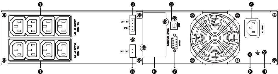
1000VA / 1500VA / 2000VA Standard & 1000VA / 1500VA Supercharger-Modell, Rückseite
