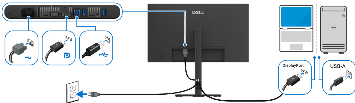
Figuur 30. DisplayPort-aansluiting
